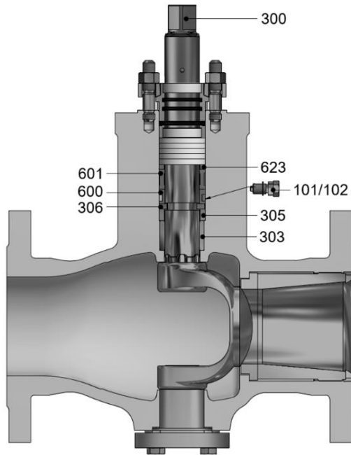
Bild 3-21: Typ 72.3, DN 100 (Stopfbuchse mit O-Ringen)
