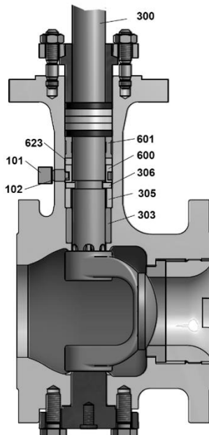
Bild 3-23: Typ 72.4, DN 100 (Stopfbuchse ohne O-Ringen)
