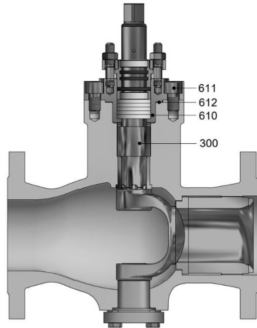
Bild 3-22: Typ 72.3-02, DN 100 (Stopfbuchse mit O-Ringen)
