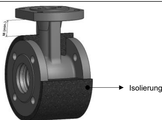
Fig. 5-2: Isolierungsgrenze · Drehkegelventil Standarddesign
