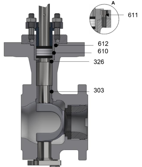
Bild 3-24: Typ 72.4-02, DN 100 (Stopfbuchse ohne O-Ringen)
