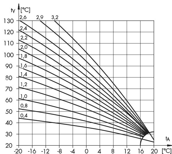
Rys. 4 - Krzywe grzania
