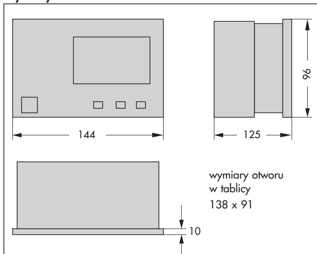
Rys. 7 · TROVIS 5479
