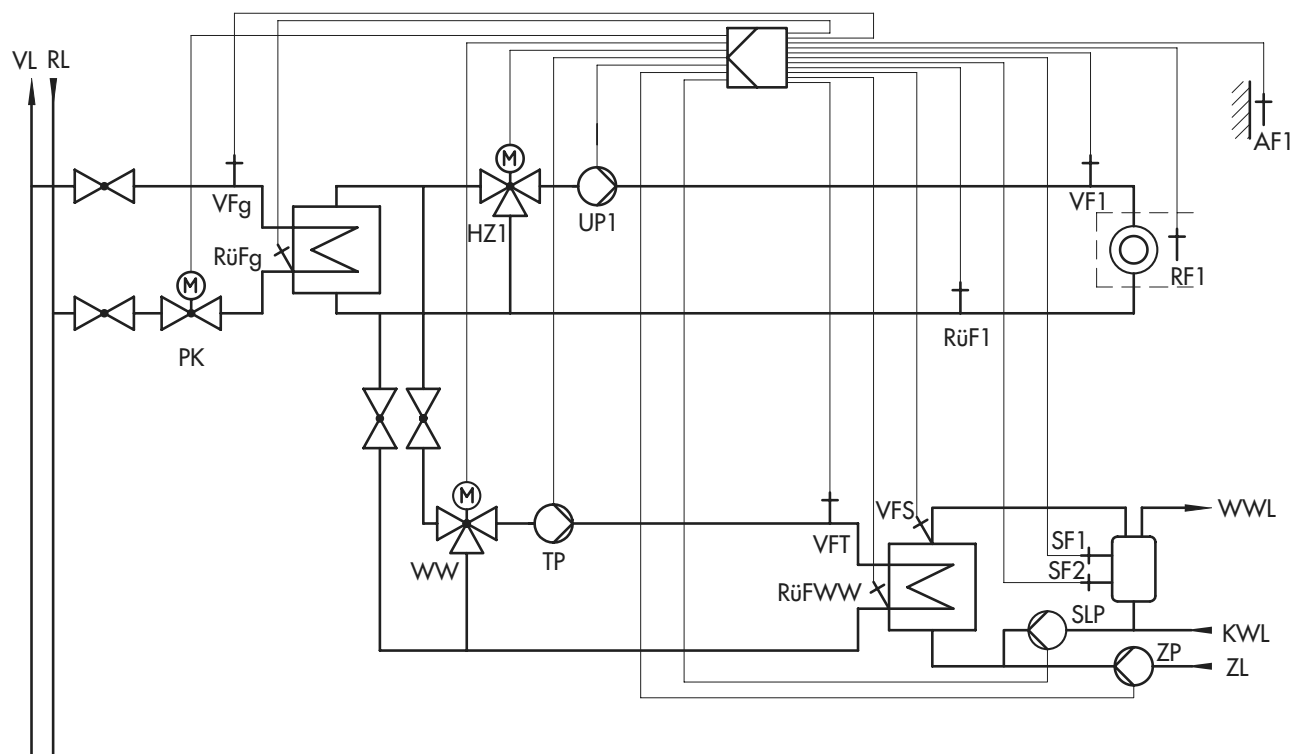
Rys. 11 · Instalacja nr 4
