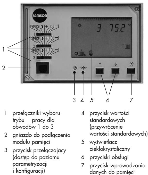
Rys. 3 · Elementy obsługi regulatora TROVIS 5479
