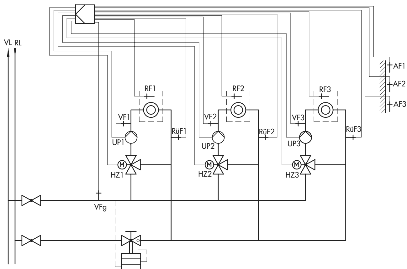
Rys. 12 · Instalacja nr 6
