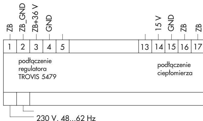
Rys. 10 · Zaciski zasilacza sieciowego dla podłączenia modułu "master" magistrali licznikowej
