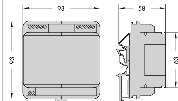
Rys. 8 · Zasilacz sieciowy dla modułu magistrali licznikowej
