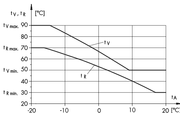
Rys. 5 - Pogodowa regulacja temperatury wody zasilającej z płynnym ograniczaniem temperatury wody powrotnej
