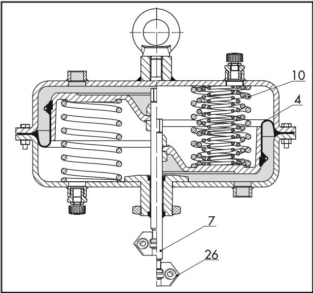
Fig. 2 : Type 3271, 1400-60 cm 2 · Sens d'action moitié gauche FE · moitié droite avec ressorts supplémentaires et sens d'action FA
