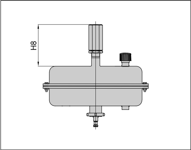
Fig. 5 : Surface du servomoteur 1400-60 cm 2 , avec limitation de course réglable
