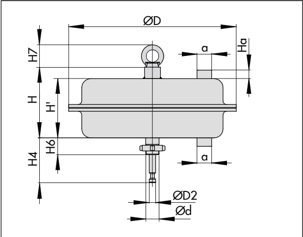
Fig. 4 : Type 3271 avec surface de 1400-60 cm 2
