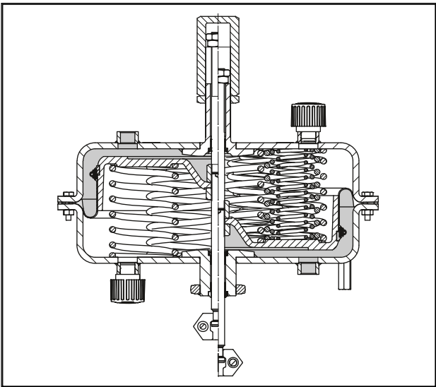
Fig. 3 : Exécution 1400-60 cm 2 avec limitation de course bidirectionnelle réglable
